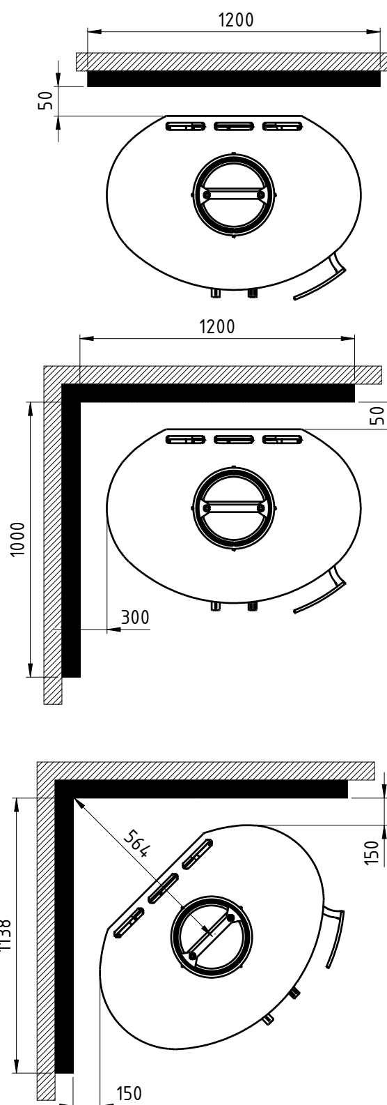
Ild 10 ECO - z szybą boczną
