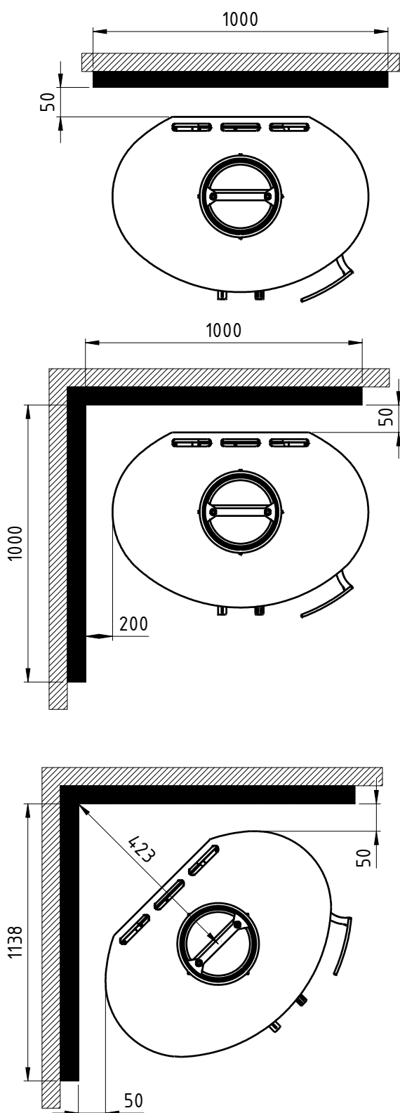
Ild 9 ECO and 11 ECO - bez szyby bocznej
